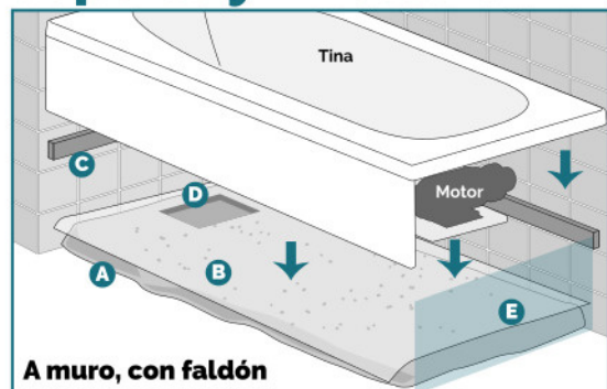
Meseta niveladora
